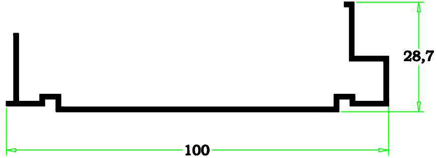
88-10 0.532 kg/m
