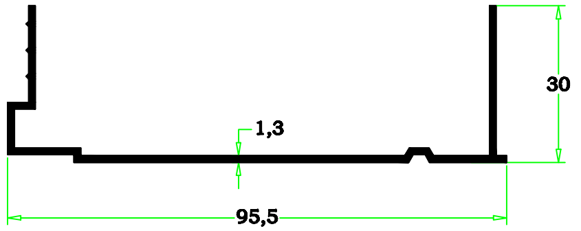
87-58 0.527 kg/m
