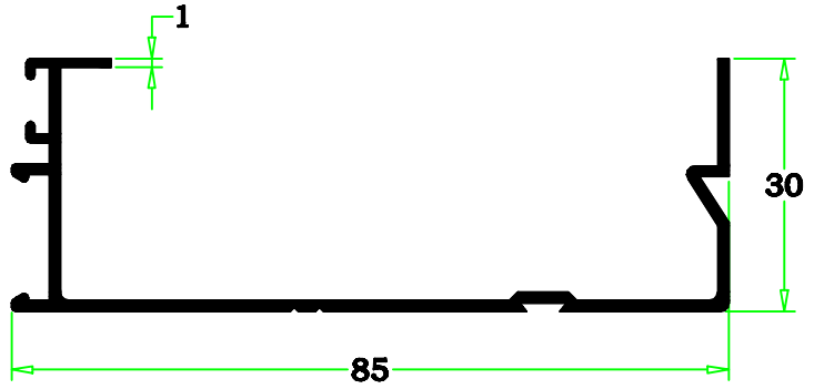
86-28 0.568 kg/m
