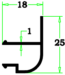
88-1 0.163 kg/m
