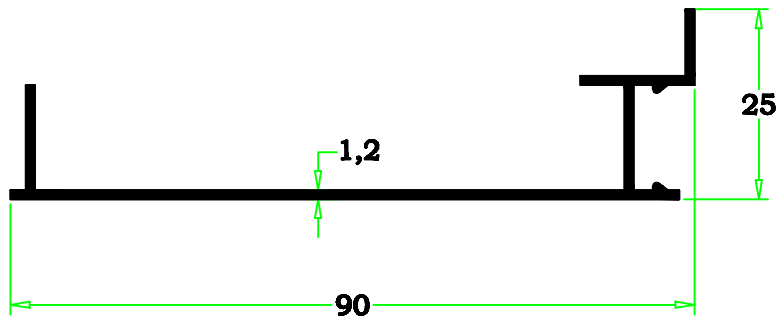
88-2 0.458 kg/m
