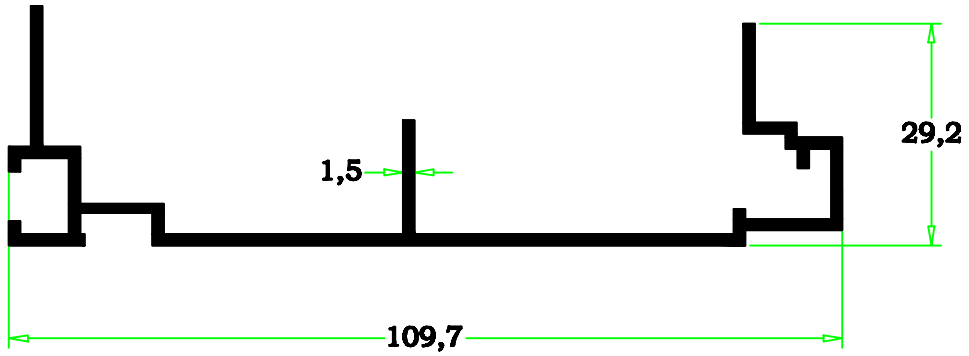
86-66 0.976 kg/m
