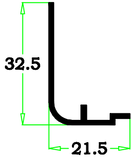
83-19 0.190 kg/m
