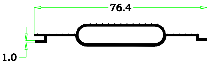
82-48 0.344 kg/m
