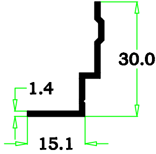
87-57 0.182 kg/m
