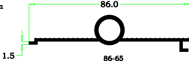
86-65 0.585 kg/m
