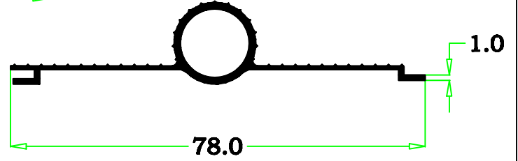
86-6 0.283 kg/m
