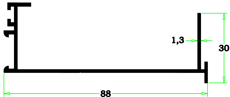
89-44 0.569 kg/m
