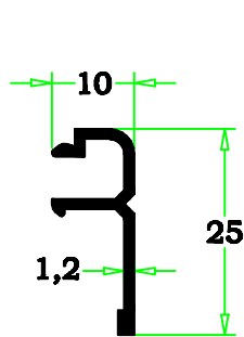
98-21 0.150 kg/m
