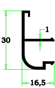
86-27 0.189 kg/m
