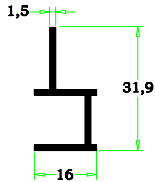
86-47 0.221 kg/m
