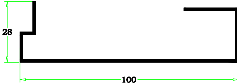
87-77 0.679 kg/m
