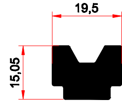
3000 0,631 kg/m
