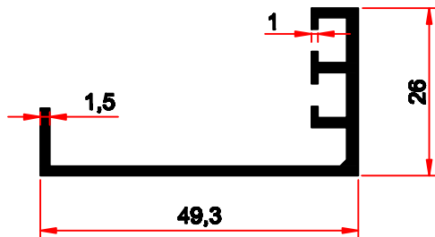
3224 0,444 kg/m
