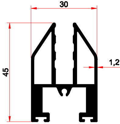
2967 0,994 kg/m
