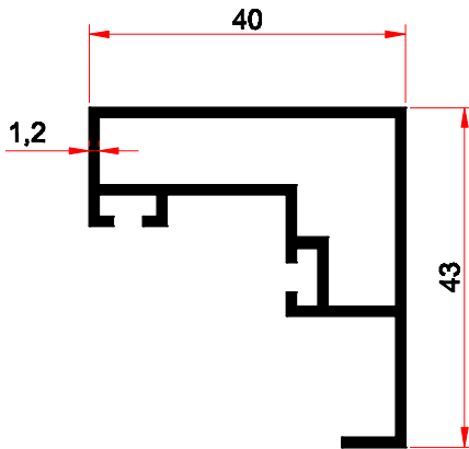
3019 0,557 kg/m
