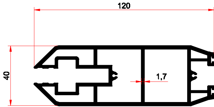
3038 2,558 kg/m
