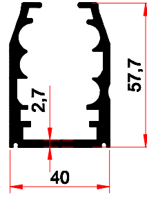
2968 1,480 kg/m
