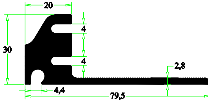
2006-115 1,558 kg/m
