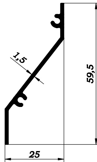
2011-33 0,333 kg/m
