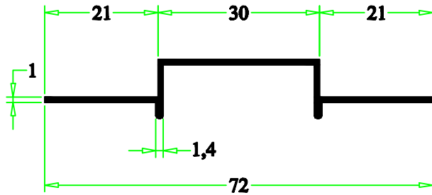
2008-40 0,255 kg/m
