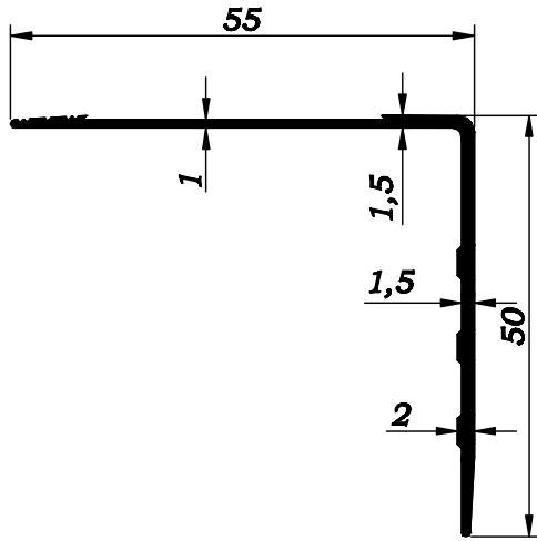
2011-13 0,369 kg/m
