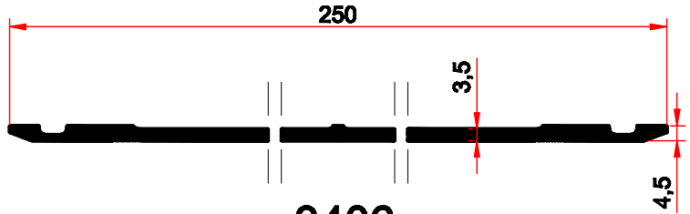
3406 2,417 kg/m
