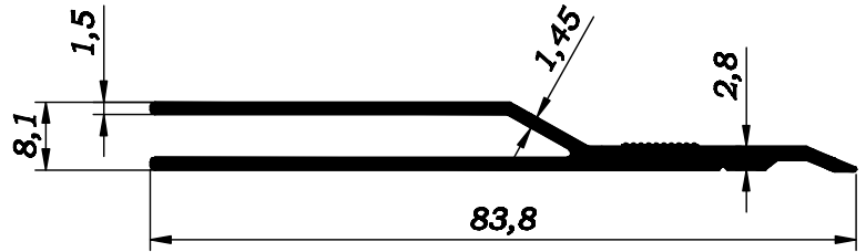
2011-23 0,639 kg/m
