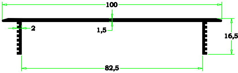
2009-02 0,526 kg/m
