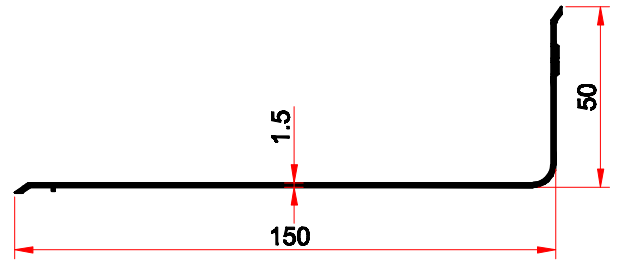
2938 0,819 kg/m
