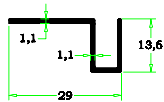
2010-103 0,161 kg/m
