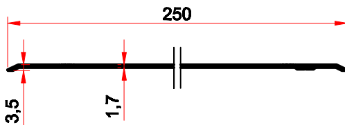
3075 1.170 kg/m
