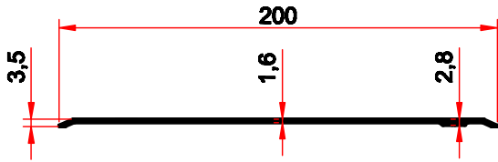
3036 0.891 kg/m
