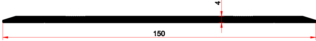
3017 1,567 kg/m
