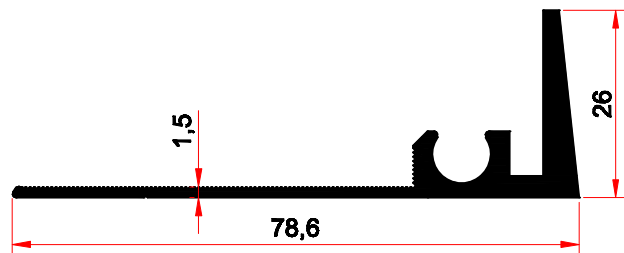
3002 0,686 kg/m
