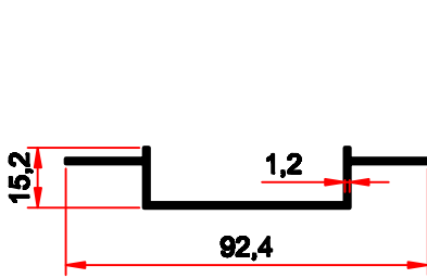
2988 0,391 kg/m
