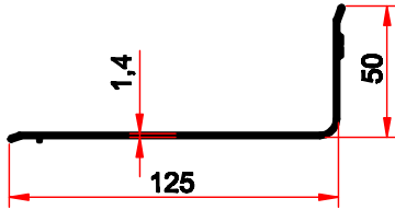
3404 0,689 kg/m
