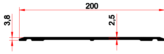
3037 1.447 kg/m
