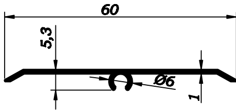
2009-87 0,189 kg/m
