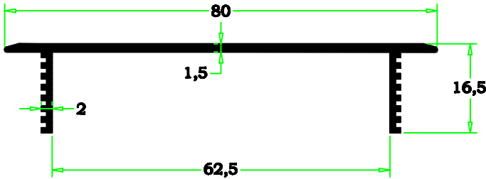
2009-03 0,445 kg/m
