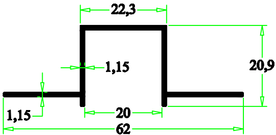
2006-113 0,316 kg/m
