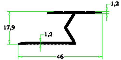
2010-01 0,231 kg/m
