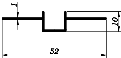
2011-32 0,189 kg/m
