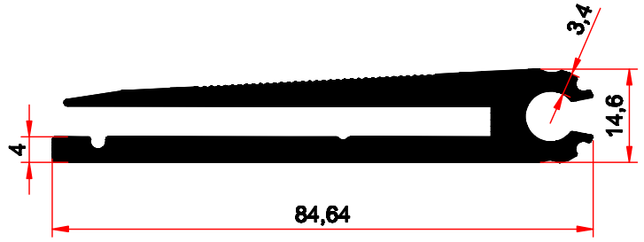
3401 1,765 kg/m
