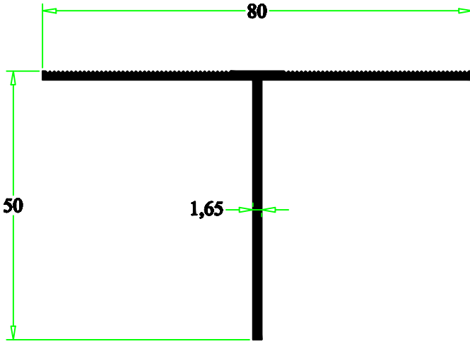
2006-119 0,537 kg/m
