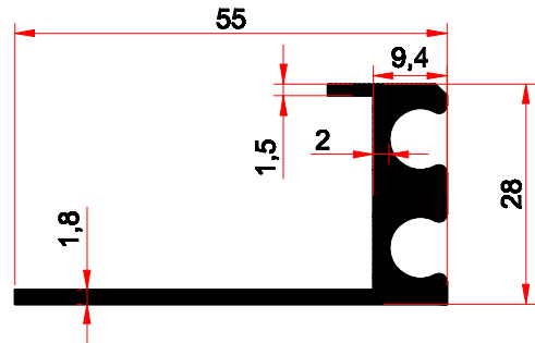
2009-29 0,683 kg/m
