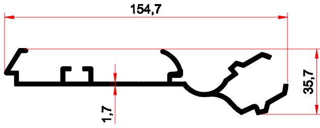
2008-21-B 1.346 kg/m
