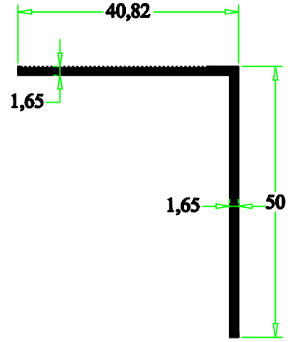
2006-118 0,380 kg/m
