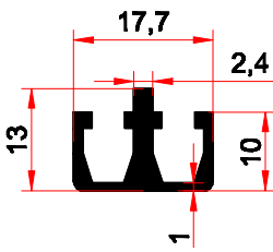
2009-28 0,230 kg/m
