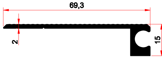
3020 0,533 kg/m
