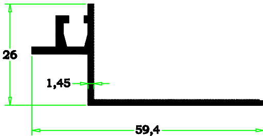
2010-32 0,374 kg/m
