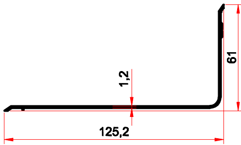
2008-47-B 0.605 kg/m
