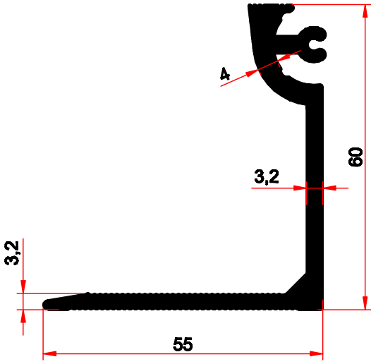
3400 1,201 kg/m
