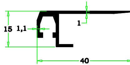
2010-93 0,229 kg/m
