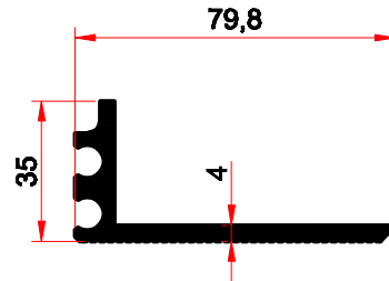
2008-45-B 1.227 kg/m
