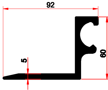
2989 2,315 kg/m
