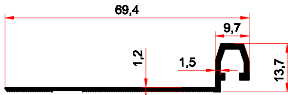
2009-30 0,295 kg/m
