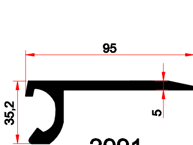
2991 1,823 kg/m
