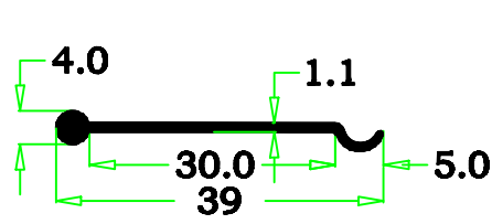
2005-114 0.141 kg/m
