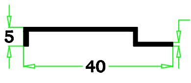
87-30 0.153 kg/m
