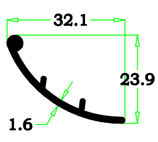
2004-112 0.226 kg/m
