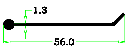
2004-36 0.230 kg/m
