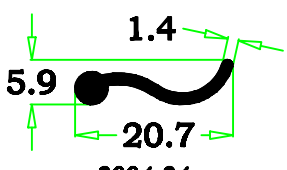
2004-24 0.114 kg/m
