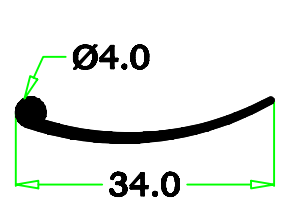
79-64 0.133 kg/m
