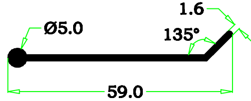
2004-59 0.298 kg/m
