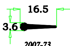
2007-73 0.081 kg/m
