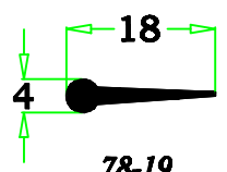
78-19 0.088 kg/m
