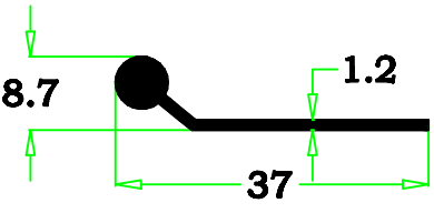
99-66 0.185 kg/m
