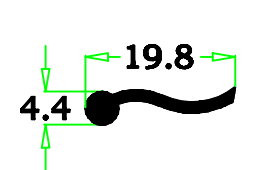
2001-67 0.102 kg/m
