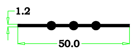
2003-59 0.225 kg/m
