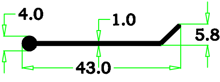
2000-93 0.144 kg/m
