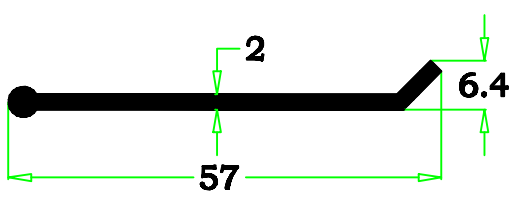
98-14 0.327 kg/m
