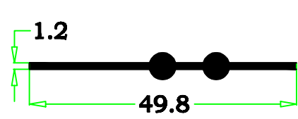
2000-30 0.235 kg/m
