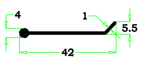
78-13 0.142 kg/m
