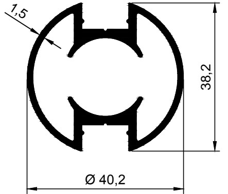
3474 0,833 kg/m
