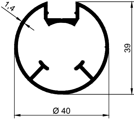
3538 0,630 kg/m
