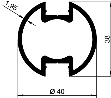
3040 0,838 kg/m
