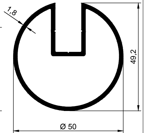
3466 0,952 kg/m
