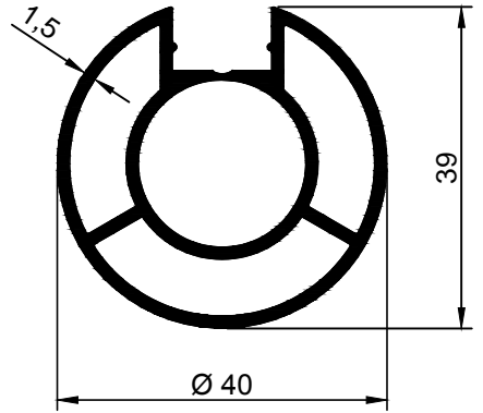
3654 0,846 kg/m
