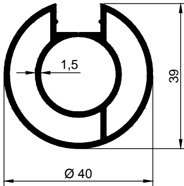
3803 0,824 kg/m
