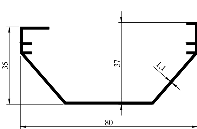
2000-55 0,464 kg/m
