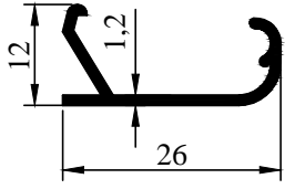
2000-138 0,158 kg/m
