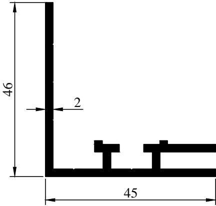
3329 0,679 kg/m
