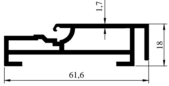
3283 0.843 kg/m
