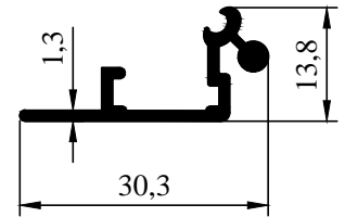
2001-111 0,207 kg/m
