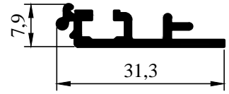
2005-71 0,193 kg/m
