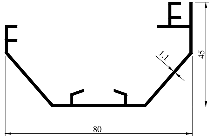
2000-59 0,554 kg/m
