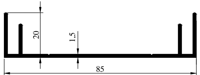
95-13 0,599 kg/m
