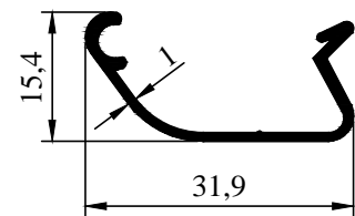
2003-116 0,184 kg/m
