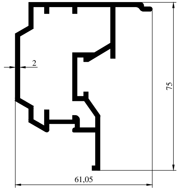
2000-149 1,450 kg/m
