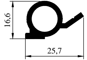
2001-2 0,340 kg/m
