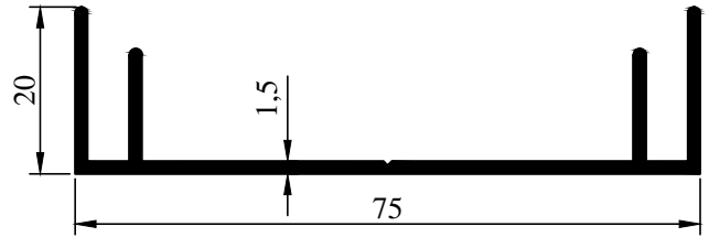
79-84 0,560 kg/m
