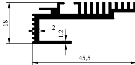
3495 0,556 kg/m
