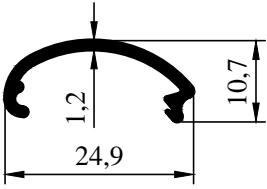
2005-68 0,128 kg/m
