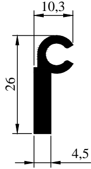
2000-134 0,325 kg/m
