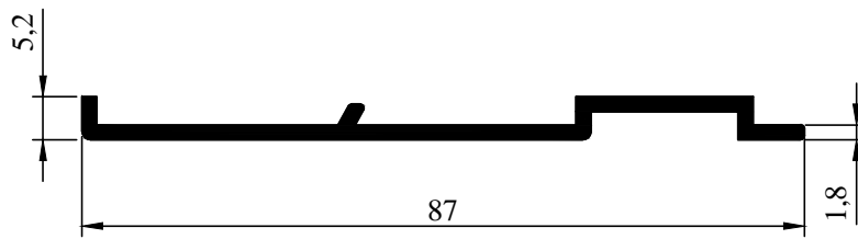
98-57 0,484 kg/m
