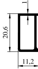
2000-135 0,162 kg/m
