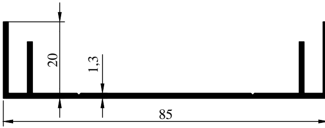
79-113 0,560 kg/m
