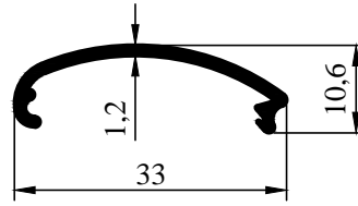
2005-70 0,151 kg/m
