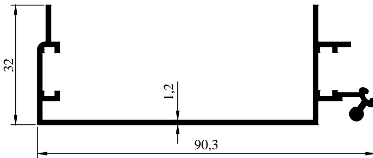
2003-115 0,626 kg/m
