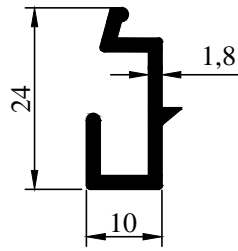
98-59 0,237 kg/m
