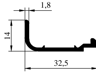
2000-4 0,203 kg/m
