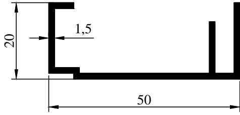
85-74 0,426 kg/m
