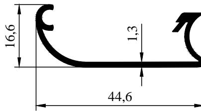
2001-110 0,160 kg/m
