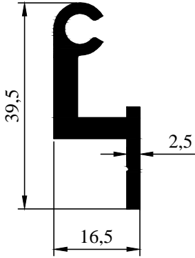
2000-133 0,555 kg/m
