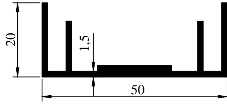
81-12 0,542 kg/m
