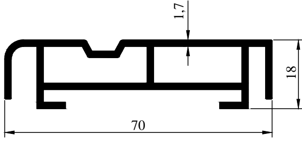
3282 0.944 kg/m
