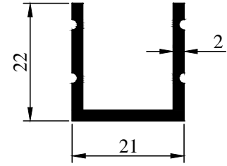
2002-85 0,346 kg/m
