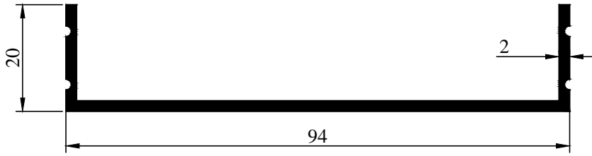
2002-84 0,719 kg/m
