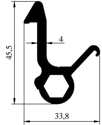
2001-1 0,874 kg/m
