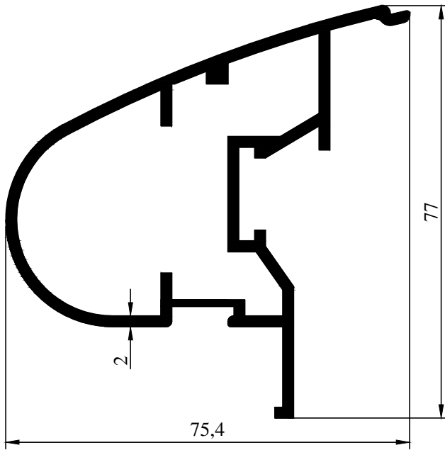
2000-148 1,496 kg/m
