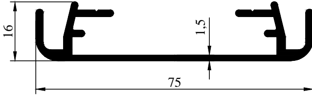
2000-2 0,727 kg/m
