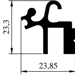
2000-137 0,441 kg/m
