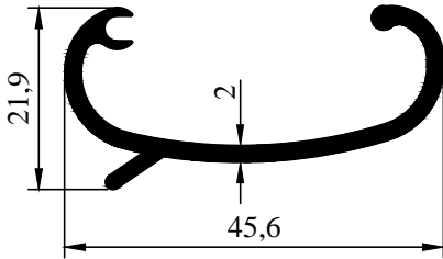
2005-127 0,453 kg/m
