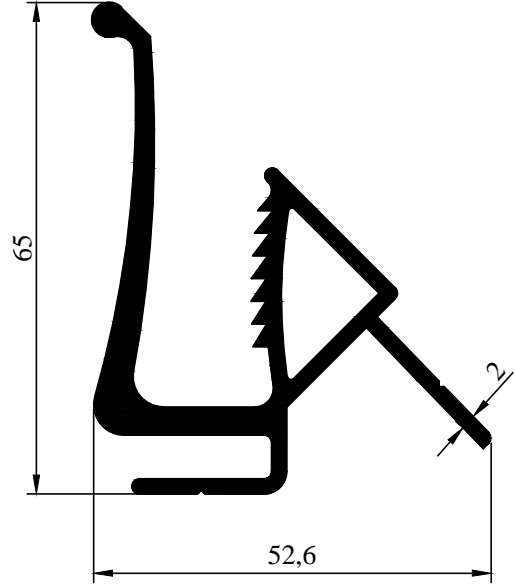
99-14 1,426 kg/m
