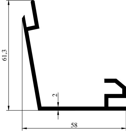
2002-76 0,813 kg/m
