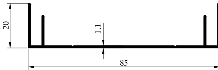
95-18 0,423 kg/m
