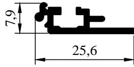
2005-69 0,160 kg/m
