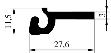
2000-136 0,310 kg/m
