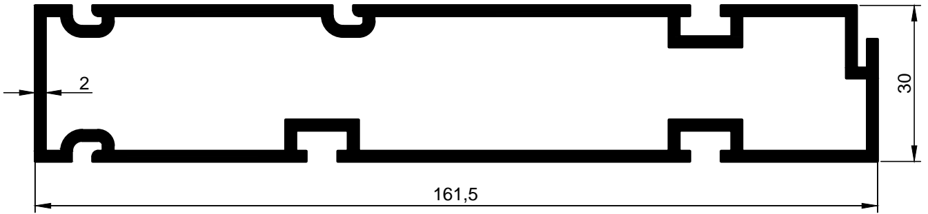
3187 2.449 kg/m
