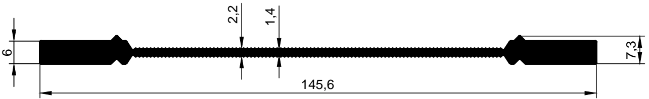
3076 1,237 kg/m
