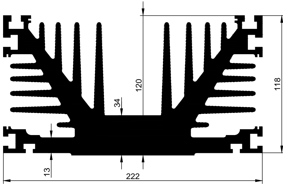
3816 32,151 kg/m
