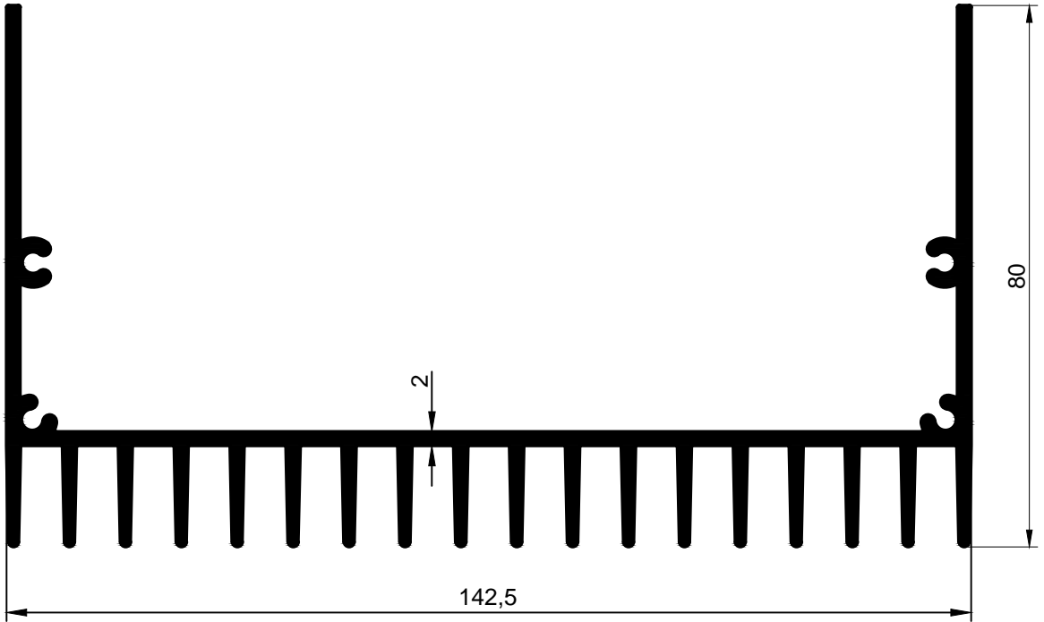
3080 2.916 kg/m
