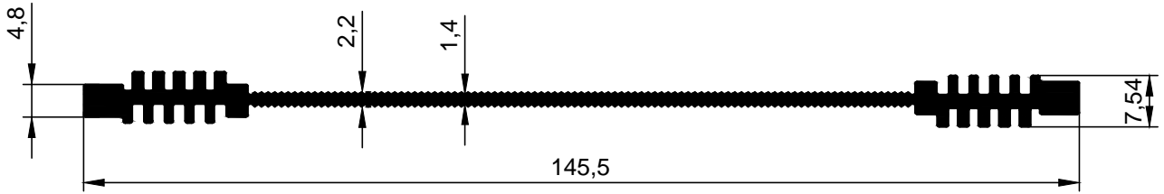
3672 1,089 kg/m
