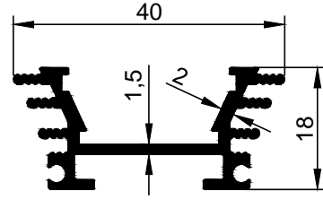
3817 0,437 kg/m
