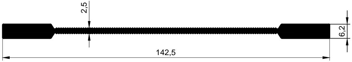
2008-50-B 1,267 kg/m
