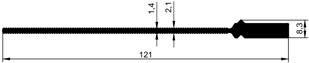
3085 0,786 kg/m
