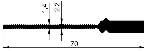
3086 0,539 kg/m
