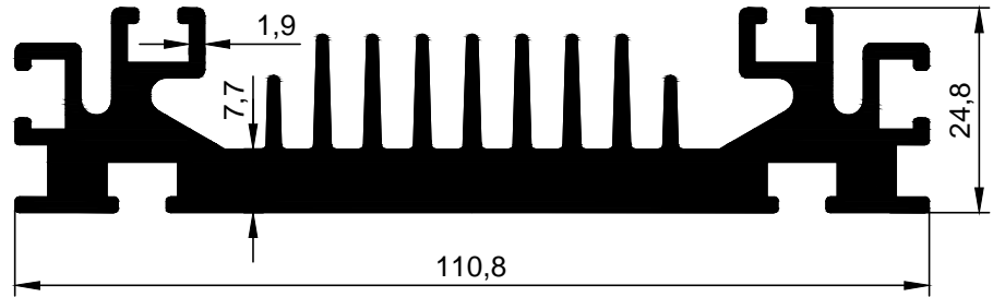
2014-121 3,483 kg/m
