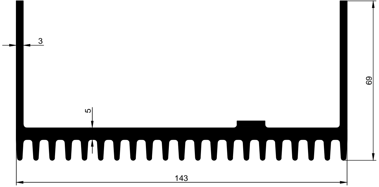
3220 4.207 kg/m
