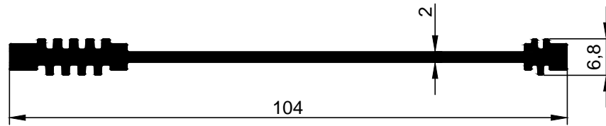
3670 0,803 kg/m
