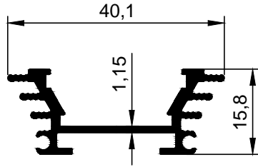
2014-117 0,349 kg/m
