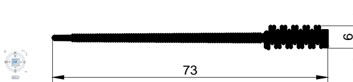
2008-34-B 0.484 kg/m
