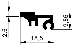
2006-123 0,223 kg/m
