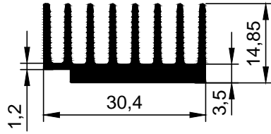
3947 0,549 kg/m
