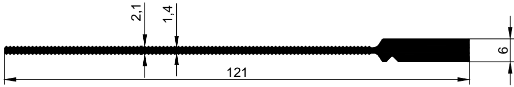
3544 0,752 kg/m
