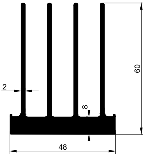
3852 2,181 kg/m
