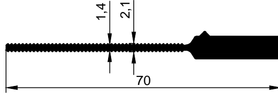
3527 0,573 kg/m
