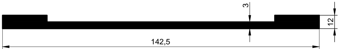
2008-51-B 1.484 kg/m
