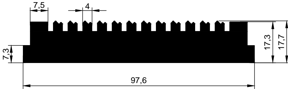
3830 4,066 kg/m
