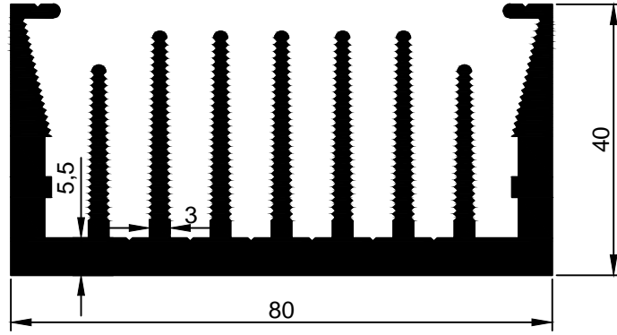
2006-121 3,465 kg/m
