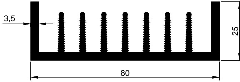
2010-08 1,853 kg/m
