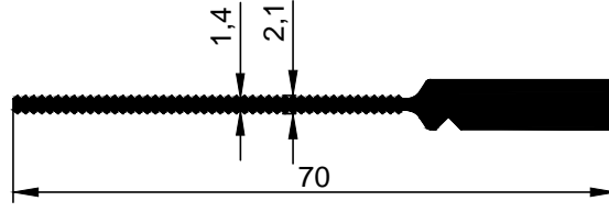
3526 0,505 kg/m
