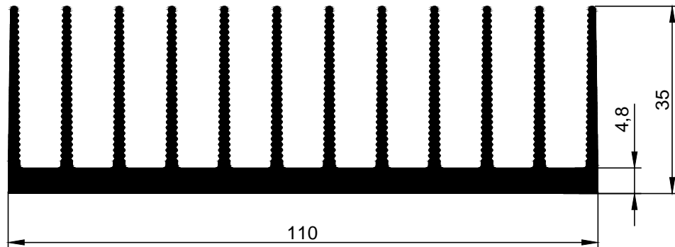
3818 3,058 kg/m
