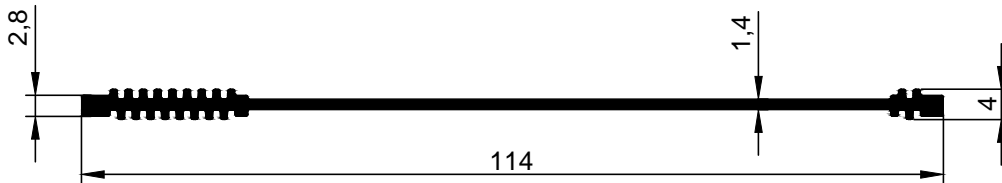
3671 0,540 kg/m
