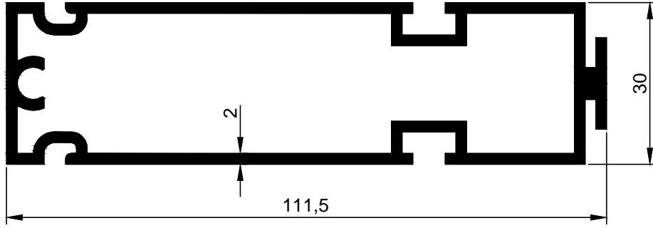
3188 1.890 kg/m
