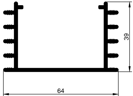
89-72 1,035 kg/m
