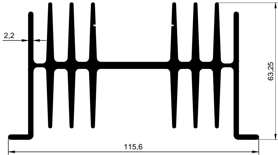
3021 3,791 kg/m
