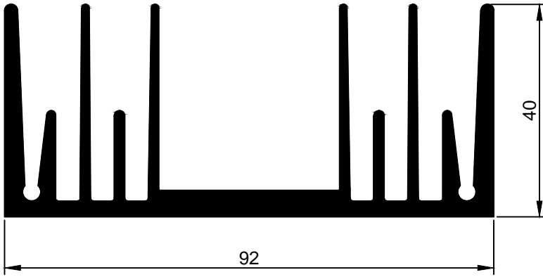
88-54 2,648 kg/m
