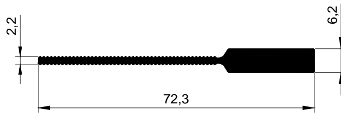
2946 0,628 kg/m
