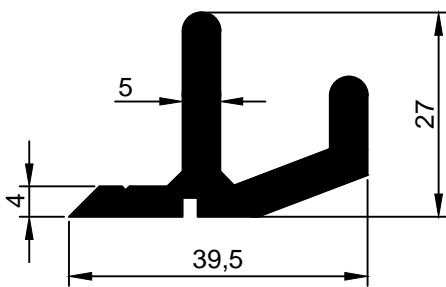
2006-122 0,876 kg/m
