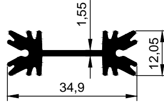
3959 0,465 kg/m
