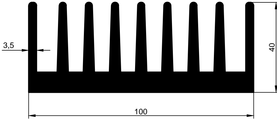
2927 5,357 kg/m
