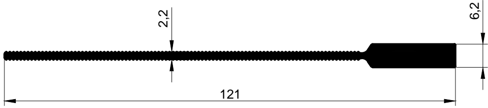
2914 0,866 kg/m
