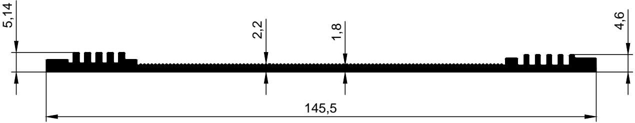
3680 0,978 kg/m
