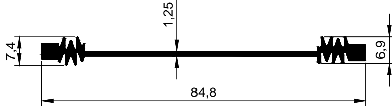
3655 0,477 kg/m
