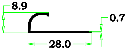
2010-50 0,088 kg/m
