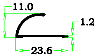
2010-64 0,090 kg/m
