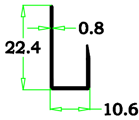
2010-60 0,093 kg/m
