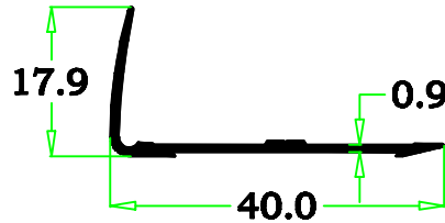
2010-77 0,153 kg/m
