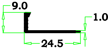
2010-53 0,102 kg/m
