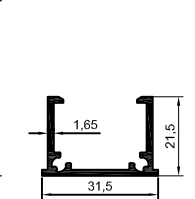
2006-117 0,363 kg/m
