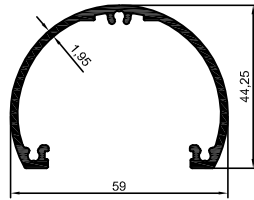
2017-40 0,790 kg/m
