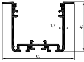
4438 1,024 kg/m
