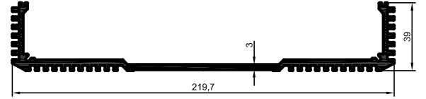
4706 3,071 kg/m
