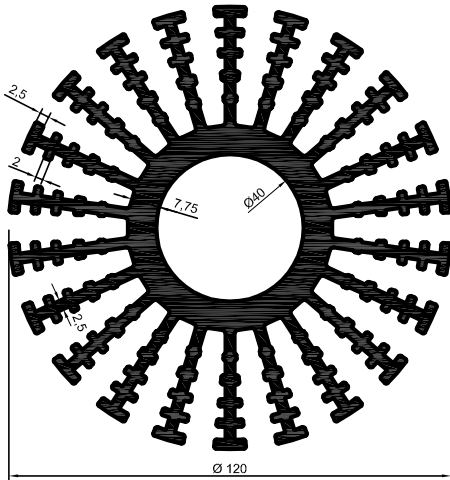
4123 10,292 kg/m
