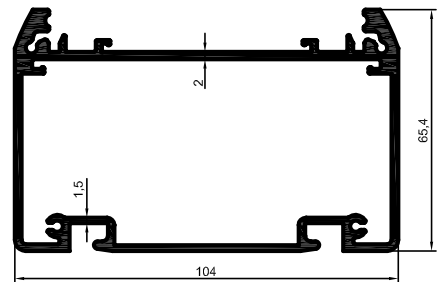
4049 2,244 kg/m
