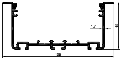
4440 1,253 kg/m
