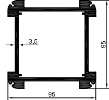
3115 4,836 kg/m
