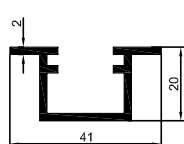
2013-40 0,482 kg/m
