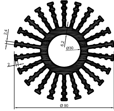
4124 6,184 kg/m
