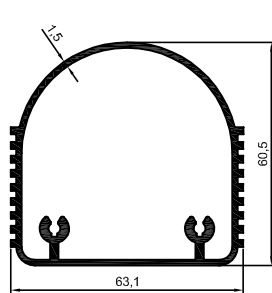
2002-137 1,224 kg/m
