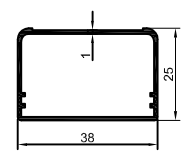
2001-86 0,342 kg/m
