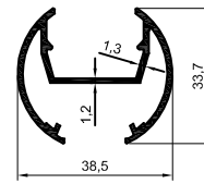
2002-73 0,483 kg/m
