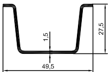
3423 0,379 kg/m
