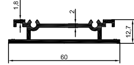
2015-03 0,755 kg/m
