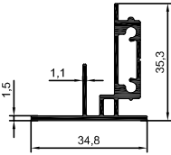
3572 0,497 kg/m
