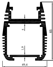
2010-90 1,960 kg/m
