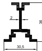
4339 0,539 kg/m
