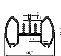
2014-115 0,801 kg/m
