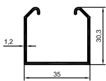
2017-08 0,343 kg/m
