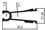
3846 0,419 kg/m
