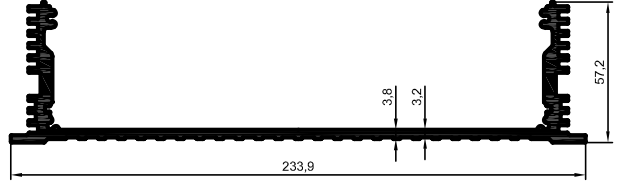
4705 3,971 kg/m
