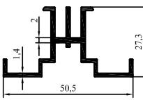
2016-34 0,558 kg/m
