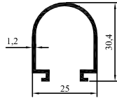
85-78 0,283 kg/m
