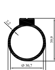
2013-10 0,815 kg/m
