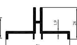
2009-37 0,538 kg/m
