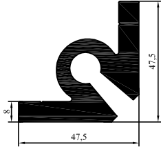
2011-54 2.466 kg/m
