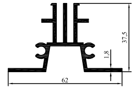
2014-106 / 4445 0,914 kg/m
