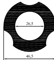
86-50 2,695 kg/m
