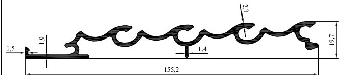
3856 1,445 kg/m
