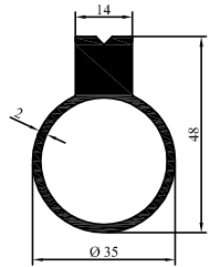
2014-03 1,062 kg/m
