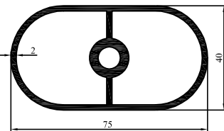
88-107 1,460 kg/m
