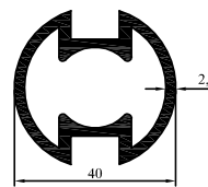
98-18 1,074 kg/m
