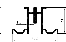
2016-27 0,483 kg/m
