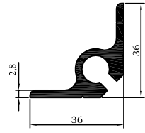
2004-92 0.766 kg/m
