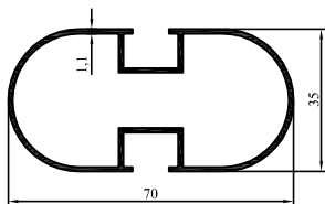
87-95 0,665 kg/m
