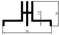
2009-36 0,735 kg/m
