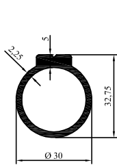
2012-42 0,653 kg/m
