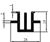
2014-107 0,428 kg/m
