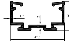
4274 0.706 kg/m
