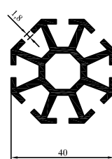
2004-137 1,228 kg/m
