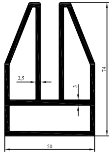
4277 2.452 kg/m
