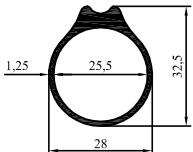
2005-90 0,427 kg/m
