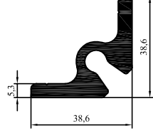
2019-01 1.210 kg/m
