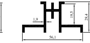
2009-93 0,710 kg/m
