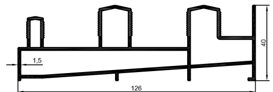
4525 1,894 kg/m
