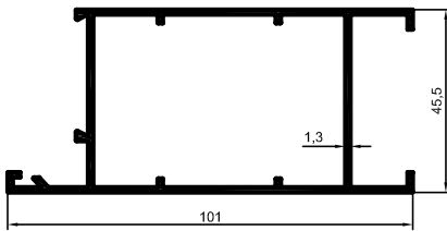
3899 1,062 kg/m
