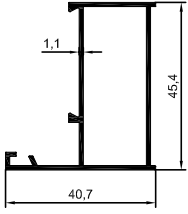
4140 0,496 kg/m
