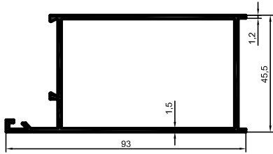
3483 1,068 kg/m
