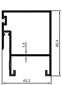
4519 0,940 kg/m
