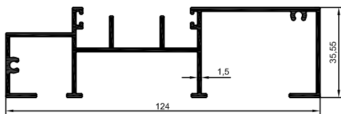
4522 1,365 kg/m
