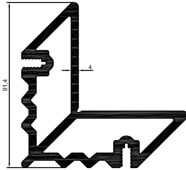
2006-59 4,446 kg/m
