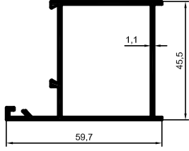
3898 0,613 kg/m
