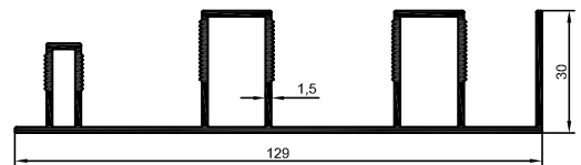
4524 1,463 kg/m
