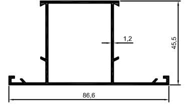
2006-149 0,780 kg/m
