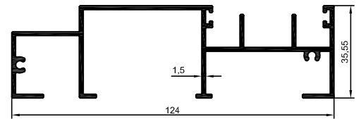
4523 1,367 kg/m
