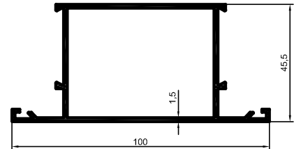
3481 1,101 kg/m
