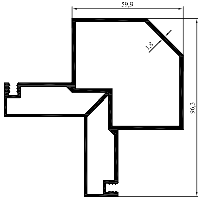
2002-190 2,025 kg/m
