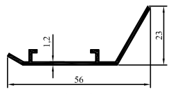
97-8 0,267 kg/m
