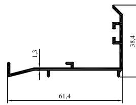
4050 0,450 kg/m
