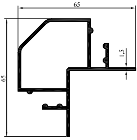
2000-153 0,952 kg/m
