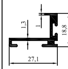
2014-88 0,290 kg/m
