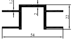
2014-124 0,541 kg/m
