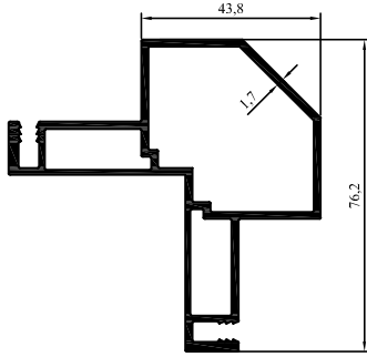
2002-188 1,447 kg/m
