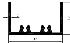
99-43 0,780 kg/m
