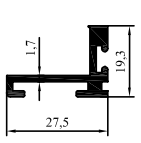
2014-44 0,353 kg/m
