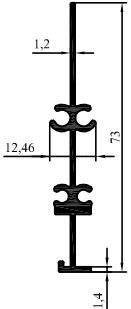
2016-29 0,481 kg/m
