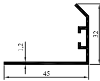
2000-17 0,294 kg/m
