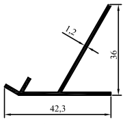
97-9 0,289 kg/m
