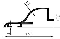
2013-30 0,271 kg/m
