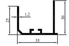
2003-102 0,313 kg/m
