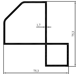
3929 1,289 kg/m
