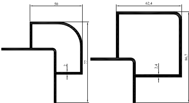
2004-99 1,276 kg/m
