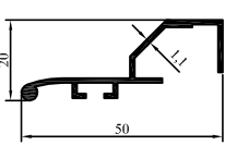
2006-07 0,308 kg/m
