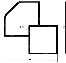
3928 0,992 kg/m
