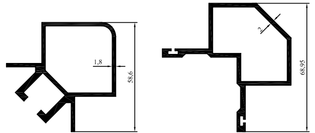
98-72 1,252 kg/m
