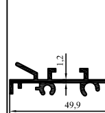
2005-18 0,502 kg/m
