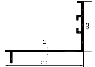
2001-28 0,582 kg/m
