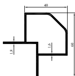
2007-89 0,802 kg/m
