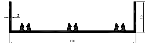
2002-4 1,270 kg/m
