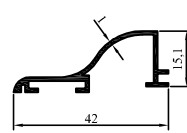
2005-113 0,238 kg/m
