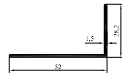
2008-86 0,319 kg/m
