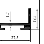
2014-43 0,293 kg/m
