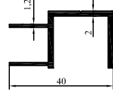
2014-125 0,449 kg/m
