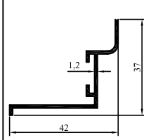
97-26 0,289 kg/m
