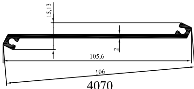
4070 0,678 kg/m
