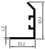
2000-16 0,238 kg/m
