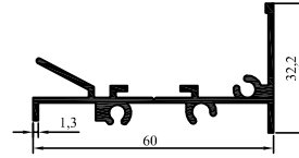
2001-63 0,618 kg/m
