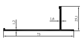
2015-77 0,350 kg/m
