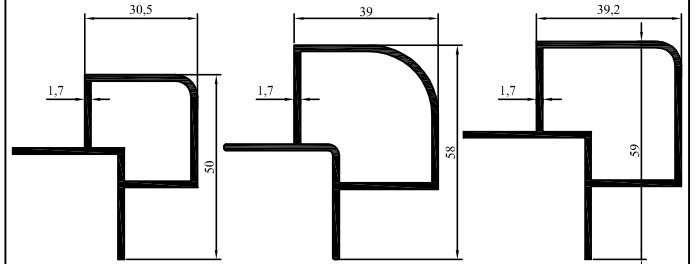
2003-86 0,697 kg/m
