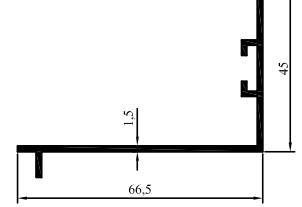
99-56 0,548 kg/m
