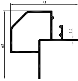
2000-154 0,869 kg/m
