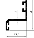
2004-154 0,281 kg/m
