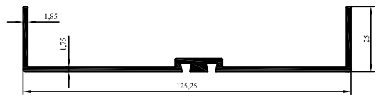
4349 0,923 kg/m
