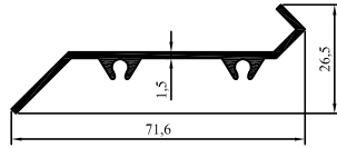
2008-85 0,468 kg/m
