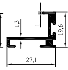
2014-50 0,300 kg/m
