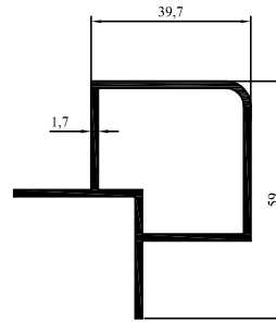
2003-31 0,864 kg/m
