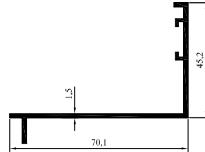
2002-97 0,569 kg/m
