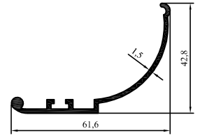
2004-113 0,459 kg/m
