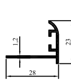
2007-65 0,199 kg/m
