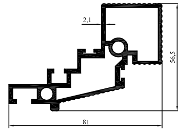
2003-139 1,614 kg/m
