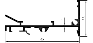
99-62 0,558 kg/m
