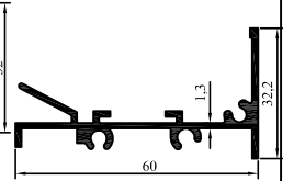
2004-26 0,625 kg/m
