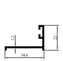
2003-166 0,222 kg/m
