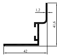
2000-94 0,303 kg/m
