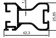
2005-140 0,569 kg/m
