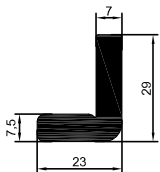
2015-29 0,854 kg/m
