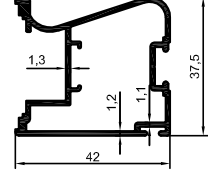
3201 0,648 kg/m
