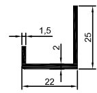
3658 0,240 kg/m
