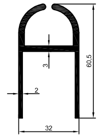
4614 1,090 kg/m
