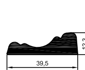
2018-09 0,771 kg/m
