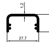
3101 0,194 kg/m
