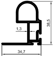
2008-38-B 0.534 kg/m
