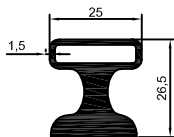
2003-182 0,844 kg/m Özen Profili
