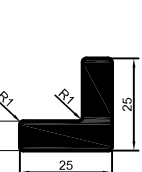
2009-99 / 4027 0,908 kg/m
