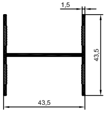
4452 0,532 kg/m
