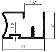
3268 0,432 kg/m
