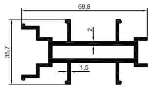
2001-58 1,134 kg/m
