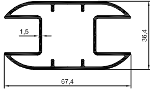
3923 1,081 kg/m
