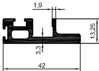
3336 0.664 kg/m
