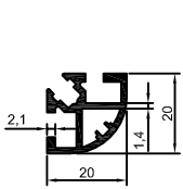
2002-37 0,351 kg/m
