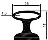
2003-181 0,786 kg/m Özel profil
