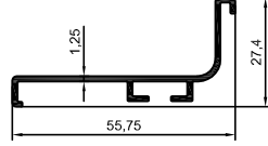
4025 0,345 kg/m
