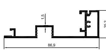
3986 0,831 kg/m
