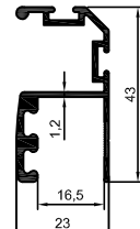
3266 0,511 kg/m
