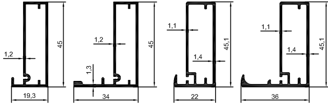
3489 0,420 kg/m 3490 0,495 kg/m 3747 0,486 kg/m 3746 0,556 kg/m
