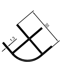
2001-118 0,420 kg/m
