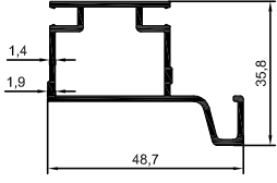
4021 0,605 kg/m
