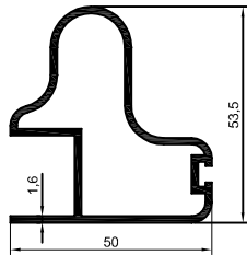
88-18 0,886 kg/m
