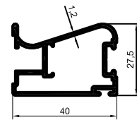
3013 0,537 kg/m
