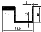
2010-107 / 3568 0,344 kg/m
