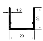
3251 0,200 kg/m
