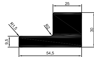
3511 2,788 kg/m
