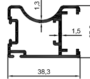
3762 0,606 kg/m
