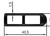
2018-41 0,542 kg/m
