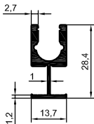
3339 0.340 kg/m
