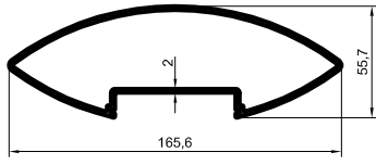
2008-74-A 2.063 kg/m
