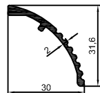
2003-180 0,253 kg/m Özel profil
