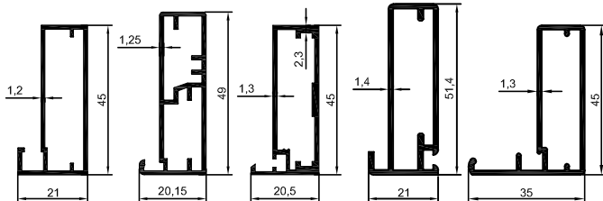
3491 0,431 kg/m 3756 0,555 kg/m 3599 0,509 kg/m 2002-124 0,585 kg/m 4500 0,522 kg/m
