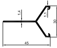
2015-52 0,288 kg/m
