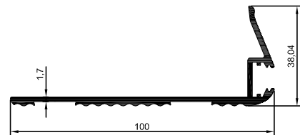
4604 0,906 kg/m
