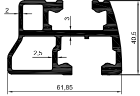
3043 2.048 kg/m
