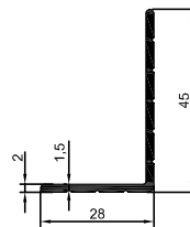
3801 0,375 kg/m
