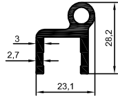
4266 0,545 kg/m
