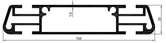
2919 2.876 kg/m
