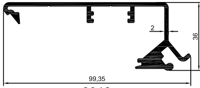
3946 1,241 kg/m
