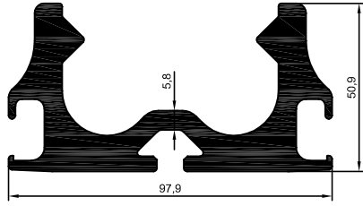
4656 4,923 kg/m
