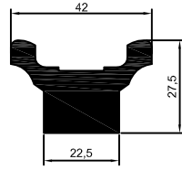
3238 1.581 kg/m
