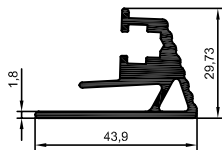
4658 0,826 kg/m
