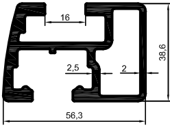
3071 1.656 kg/m
