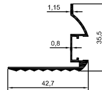
2015-68 0,350 kg/m
