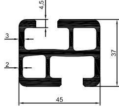
3767 1.666 kg/m
