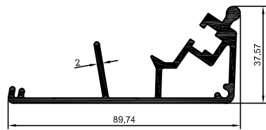
4659 1,361 kg/m
