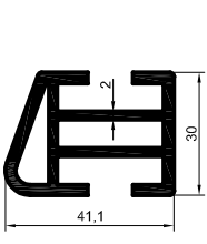
3069 1.114 kg/m
