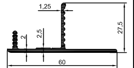
3796 0,505 kg/m
