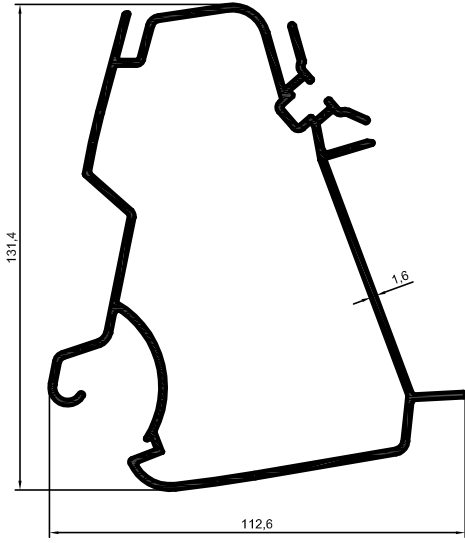
3662 2,224 kg/m
