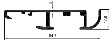
3936 0,962 kg/m
