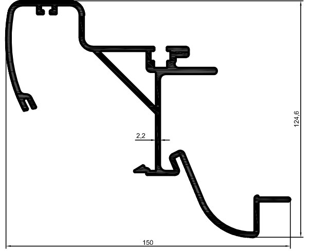
3937 3,093 kg/m
