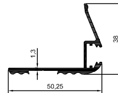
3745 0,502 kg/m
