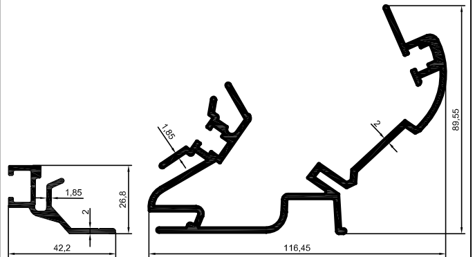
3787 0,533 kg/m
