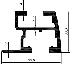
3755 1.401 kg/m
