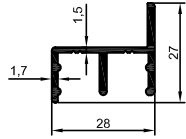
4268 0,363 kg/m
