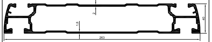
2918 4.345 kg/m
