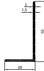
3795 0,428 kg/m
