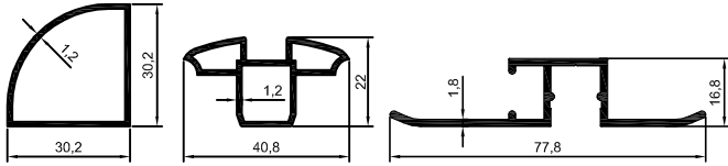
2007-84 0,343 kg/m
