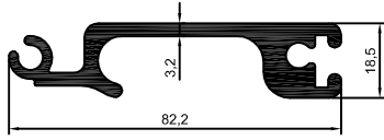
2007-53 1,492 kg/m
