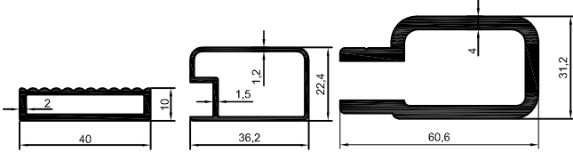
2007-78 0,468 kg/m
