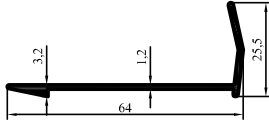
2009-88 0,315 kg/m
