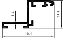
2007-29 0,405 kg/m
