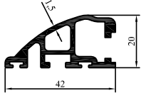
2007-01 0,606 kg/m
