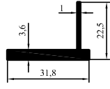
2009-89 0,362 kg/m
