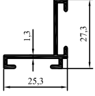
2007-28 0,255 kg/m
