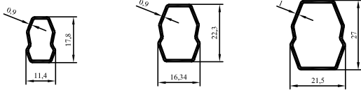
2015-60 0,119 kg/m
