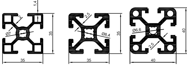
2008-19 0,998 kg/m 2006-77 1,308 kg/m 2903 1,621 kg/m
