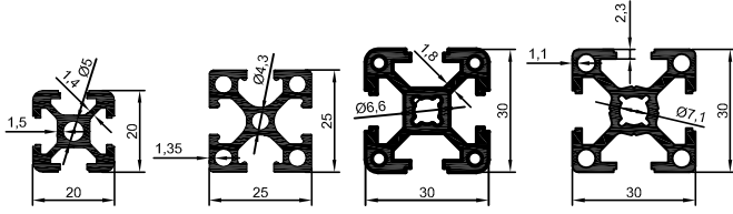
3558 0,459 kg/m 4155 0,665 kg/m 2904 0,886 kg/m 2006-89 0,833 kg/m
