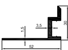
2006-74 0,548 kg/m
