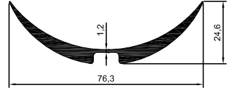
2014-42 0,890 kg/m
