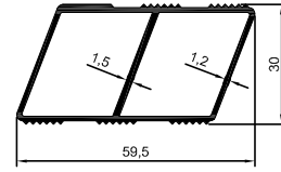
2012-16 0,702 kg/m
