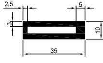
3603 0,650 kg/m
