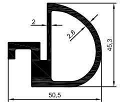
4513 1,456 kg/m
