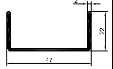
86-73 0,379 kg/m
