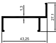
88-40 0,298 kg/m
